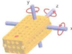
Рис. 18. Блок ЦМ-15 с 5 позициями вращения
