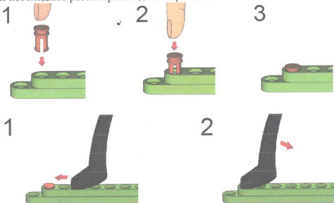
Рис. 17. Основные правила соединения деталей и демонтаж конструкции при использовании разделителя
